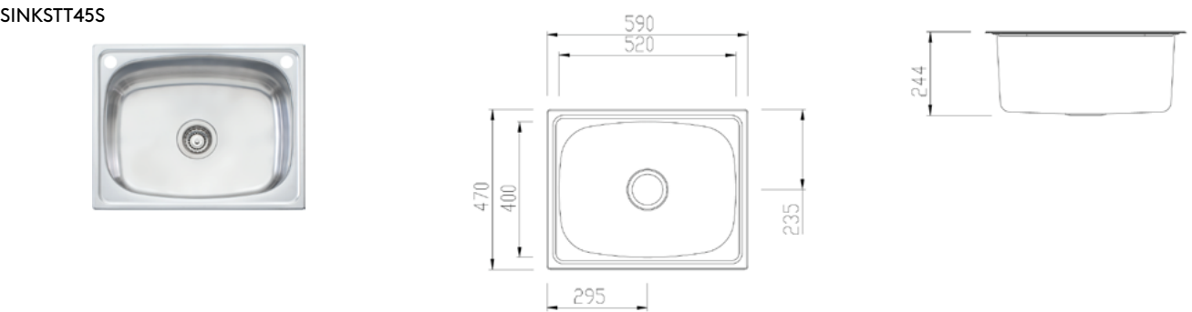
SINKSTT45S
